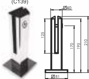
PINÇA ECO VIDRO 10mm (C139)
