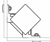
TORRE DE CANTO VIDRO 10/12/16/20mm (03)
