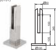
PINÇA QUADRADA MACIÇA VIDRO 10/12/16mm (C131)
